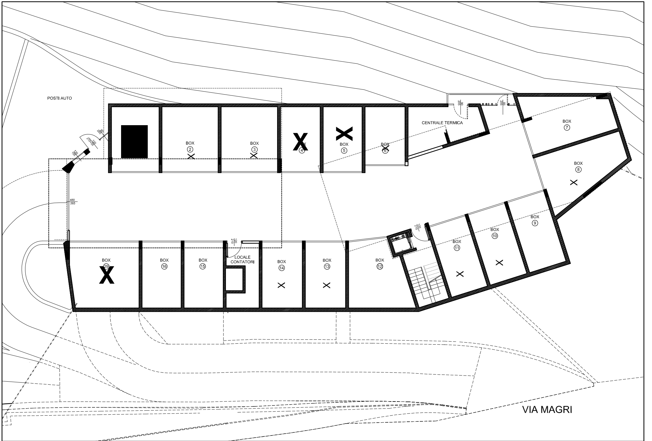
PIANO INTERRATO -2 scala 1:200
